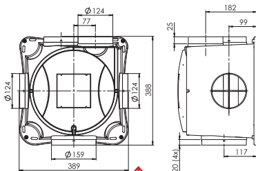
Aanzicht P ↑
