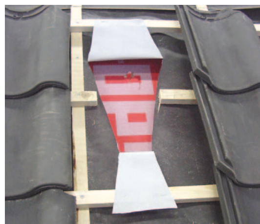
Insnijden dampdoorlatende laag Voorbeeld: 2-pans
