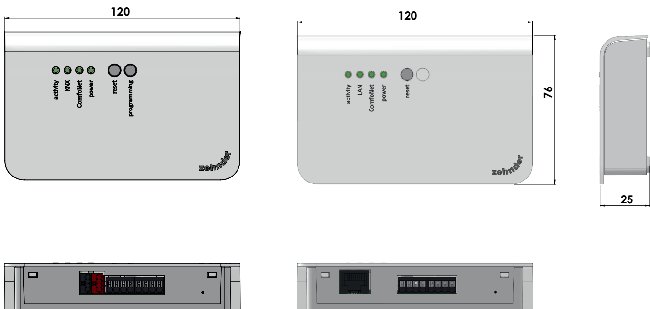
Afbeelding 3.0: Maatschets
