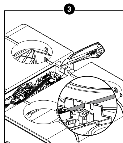
Snij één of meerdere van de voorziene stukjes uit de behuizing weg om kabels volgens het bekabelingsschema aan te sluiten.
