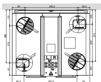
Bovenaanzicht
