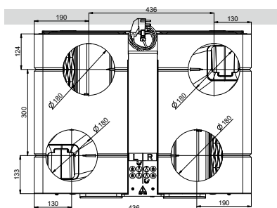
Bovenaanzicht
