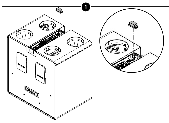
D400 en Plus-varianten: Haal de transformator uit de aftakdoos en plaats hem rechtstreeks op de voorziene plaats op de printplaat.
