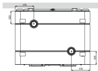
Onderaanzicht
