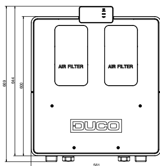
Vooraanzicht
