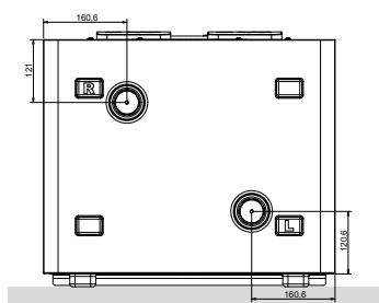
Onderaanzicht
