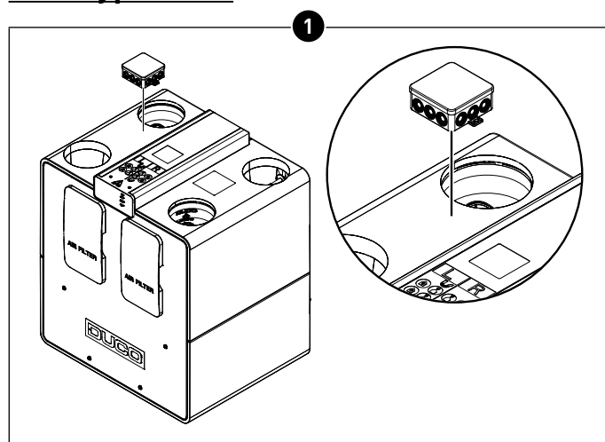
D250: monteer de aftakdoos met de transformator op het toestel naast de displaymodule.
