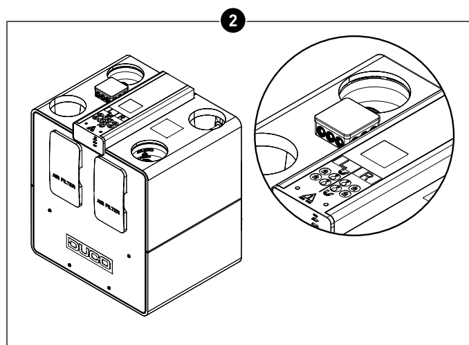
D250: Gemonteerde aftakdoos met transformator naast displaymodule.
