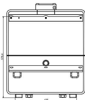
Achteraanzicht
