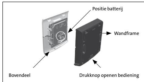
Fig. 5 Exploded view afstandsbediening 15RF
